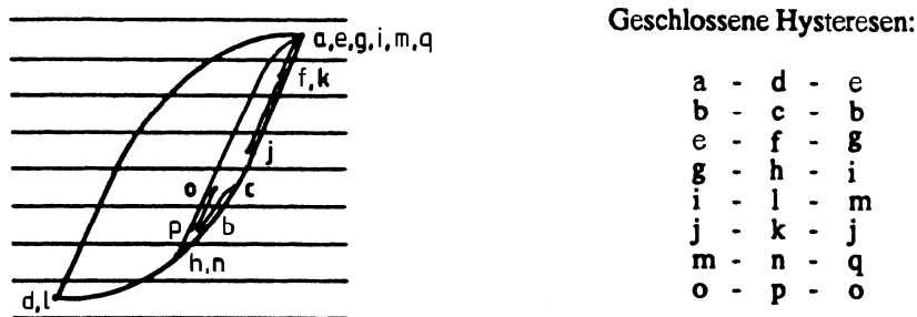
Bild 3.20: Geschlossene Hysteresen für die Beispiel-BZF
