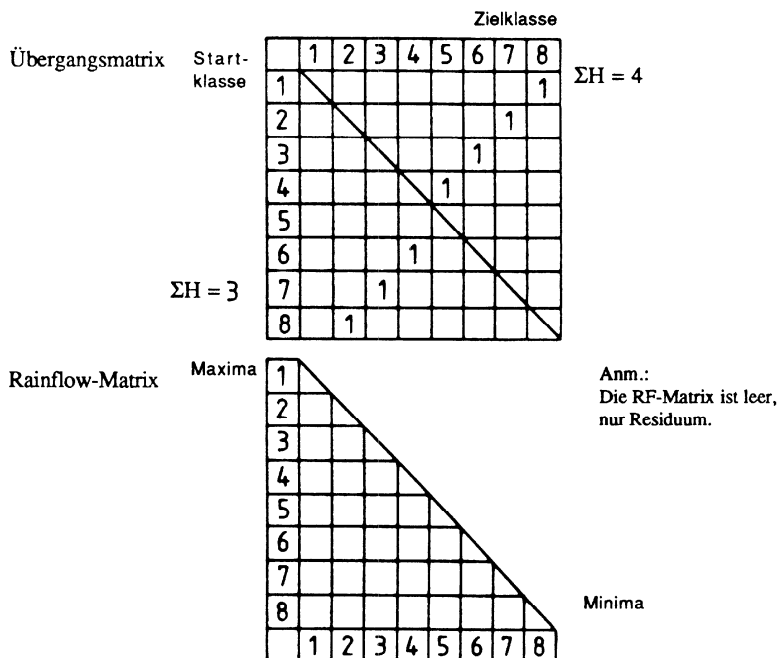
Bild 5.7: KGÜZ, BPZ, Übergangs- und Rainflow-Matrix für eine Walzstichbeanspruchung
