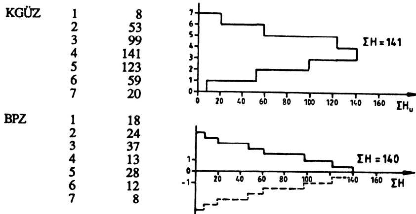
Bild 5.2: Randombeanspruchung mit I = 0,99
