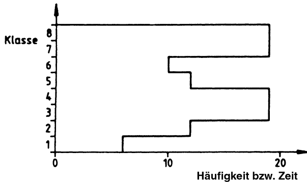
Bild 6.4: Zählergebnis Momentanwertzählung
