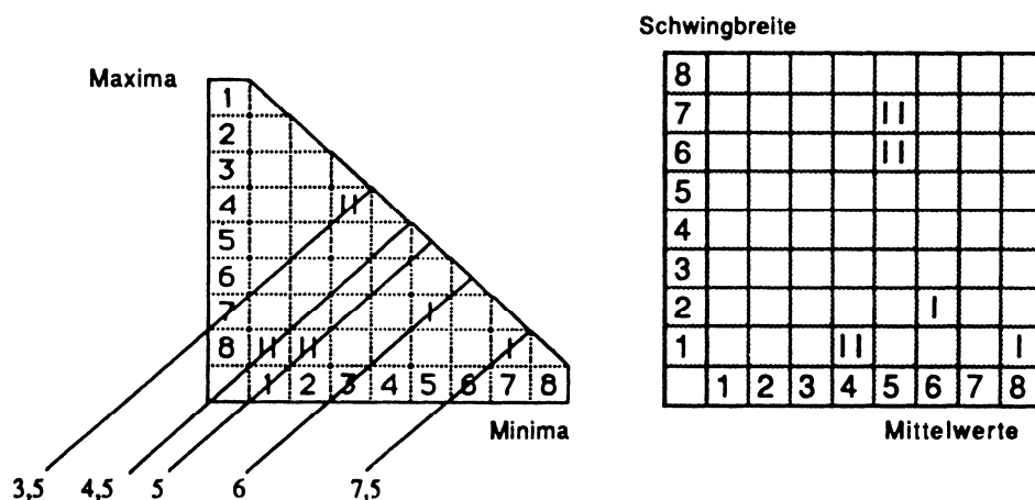
Bild 4.20: Rainflow-Matrix und die darin enthaltenen Mittelwerte der Bereichspaare
