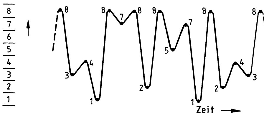
Bild 3.15: BZF Übergangsmatrix
