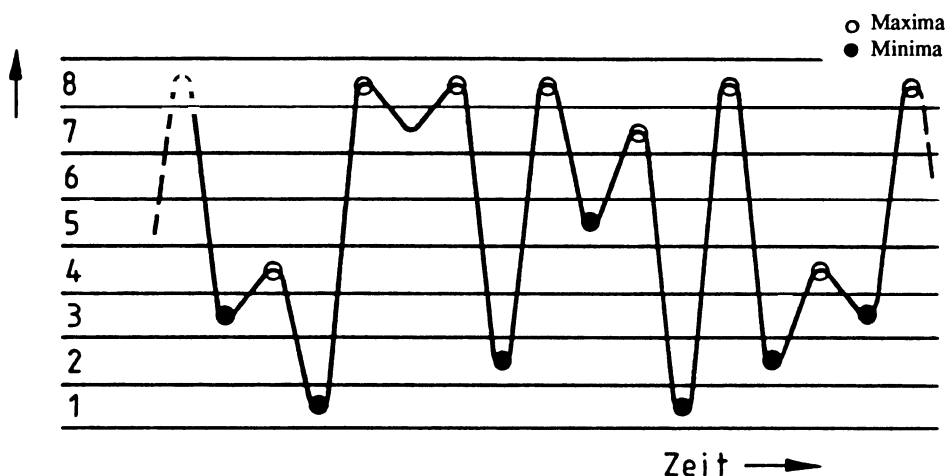
Bild 3.5: BZF Spitzenzählung
