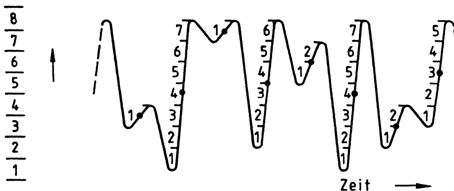
Bild 3.13: BZF Bereichs-Mittelwert-Zählung
