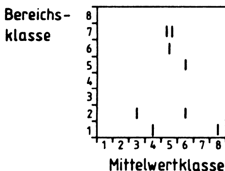
Bild 3.14: Zählergebnis Bereichs-Mittelwert-Zählung
